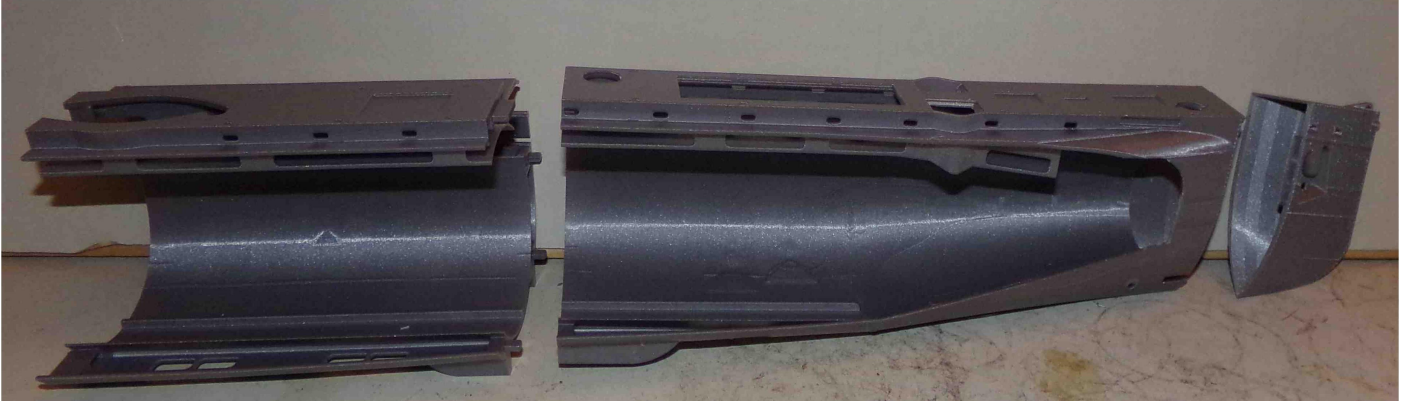
Vorderer Aussen-Rumpf: 3 Teile
